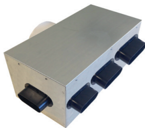
1 Plénum 5 piquages extraction / insufflation Raccord Ø 125 mm PLI 50/5P 810 510
