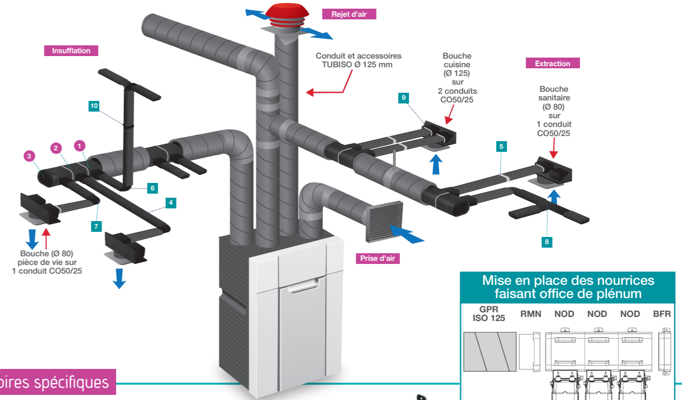
2 Nourrice modulaire Raccord conduit circulaire Ø 125 mm Permet de raccorder une bouche sur le réseau principal - Emboîtables entre elles, les nourrices font offices de plénum NOD50 810 406
